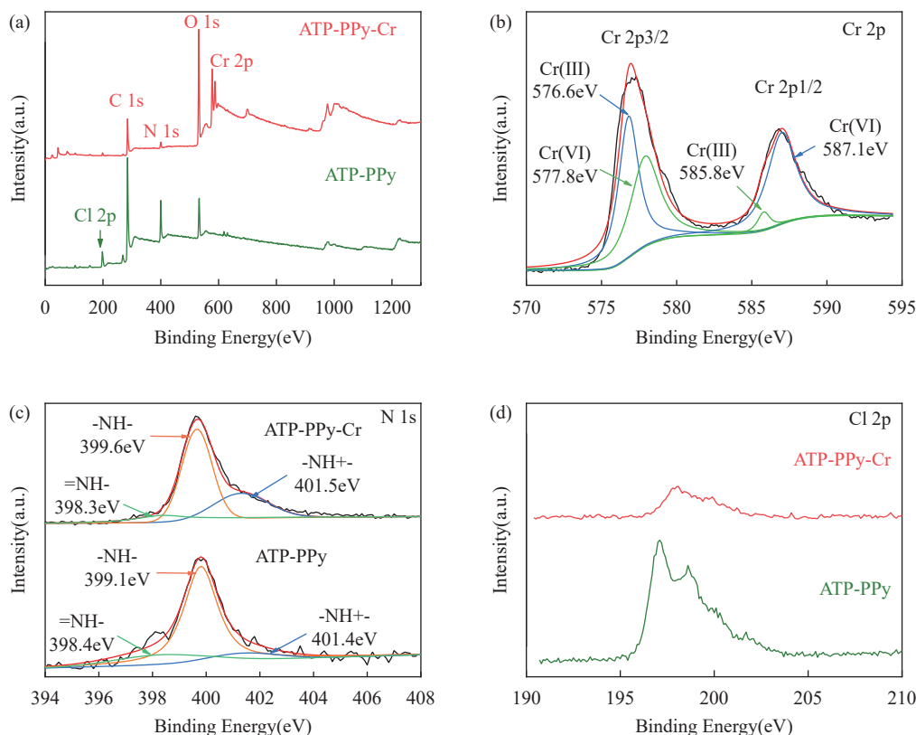
图5 XPS 光谱分析: (a) ATP/PPy 吸附 Cr(VI) 前后的宽扫描 XPS 光谱; (b) Cr 2p 光谱; (c) N 1s 谱; (d) Cl 2p 光谱
